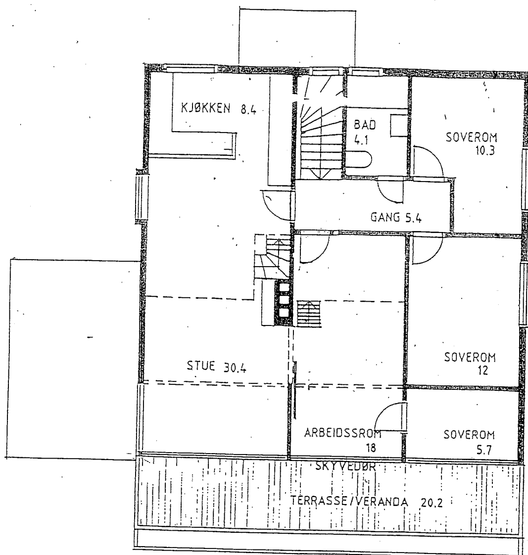
PLAN AV 2. ETASJE
