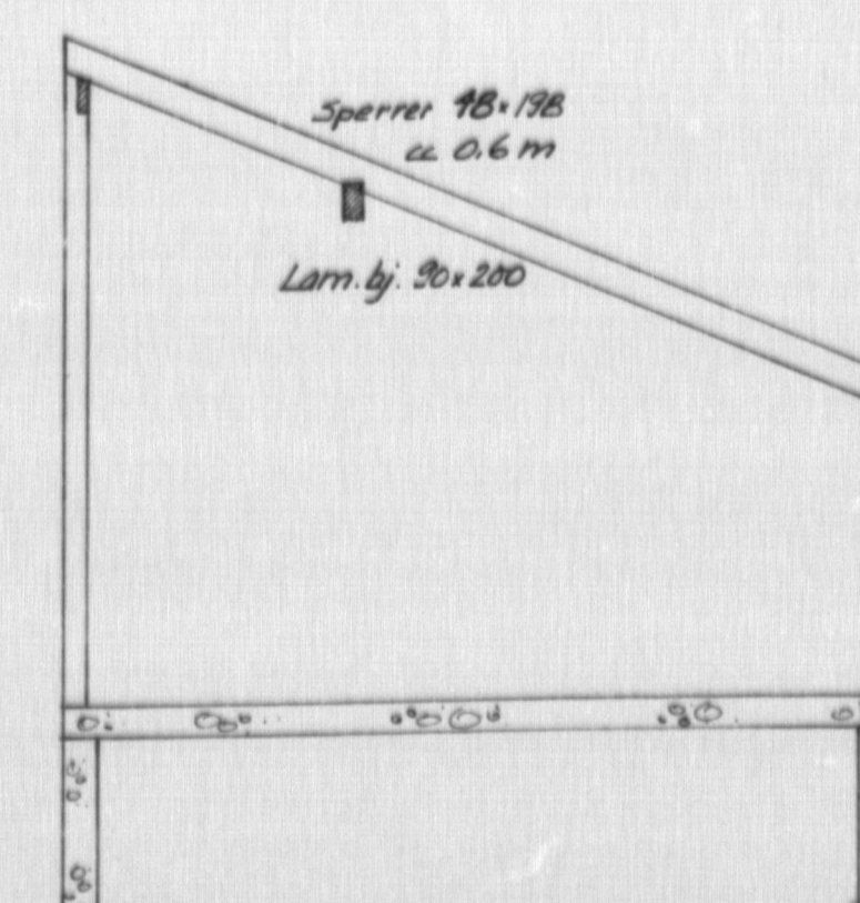
SNITT C
