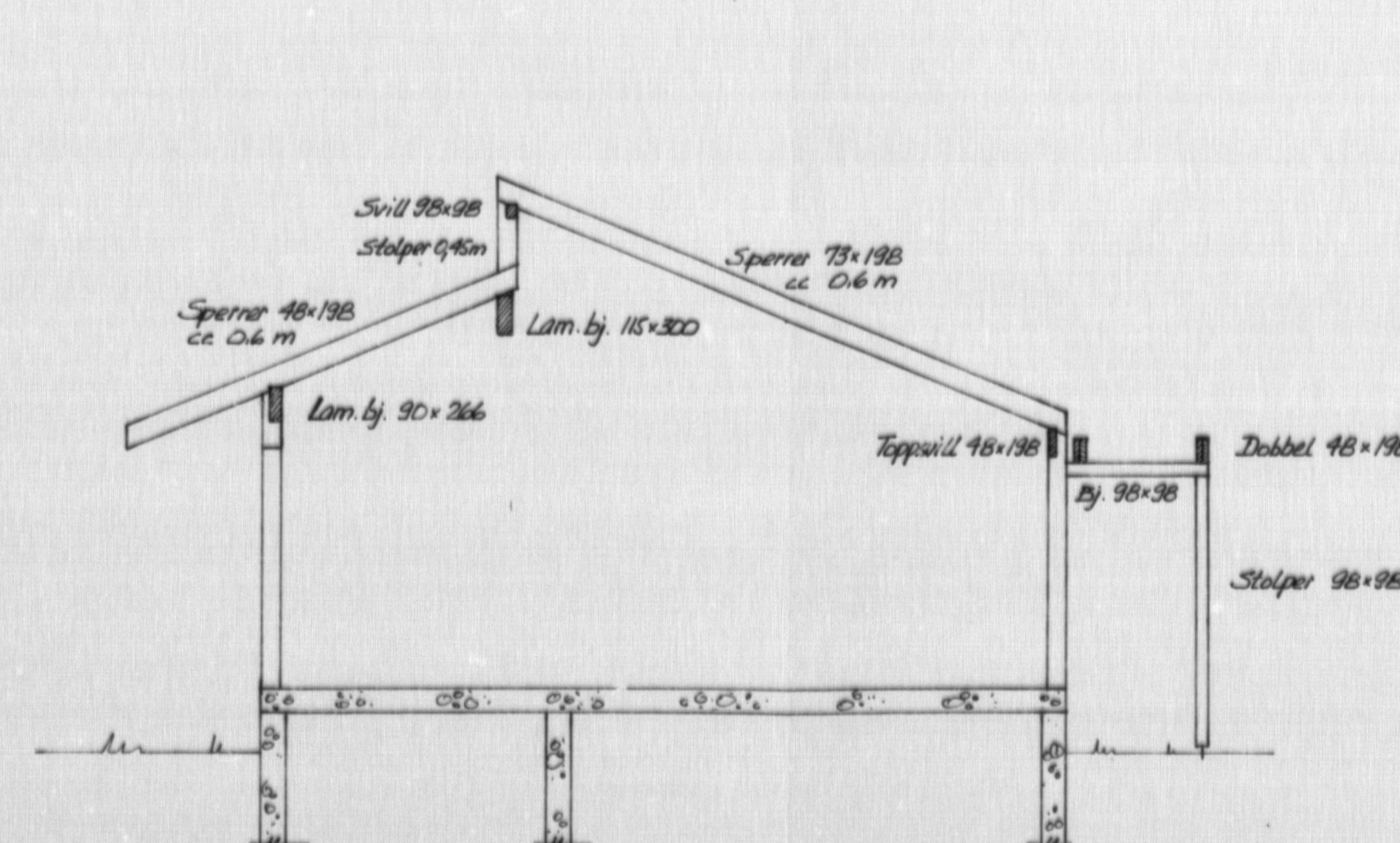
SNITT A
