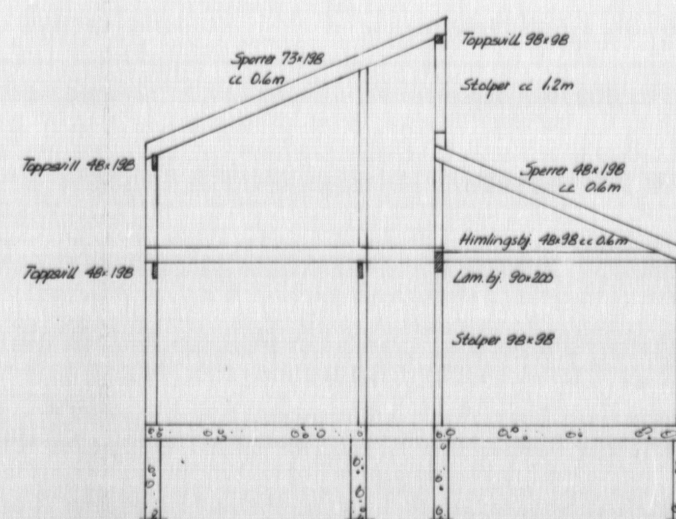
SNITT B
