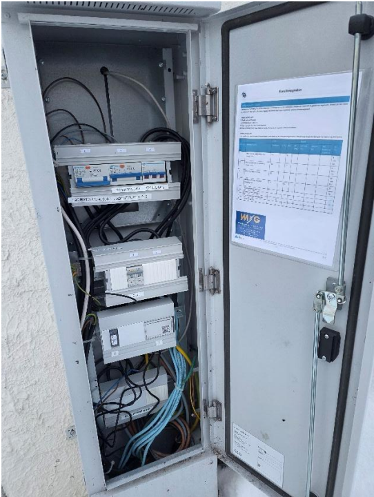
Figur 5 Sikringskap ute foran LT3.
