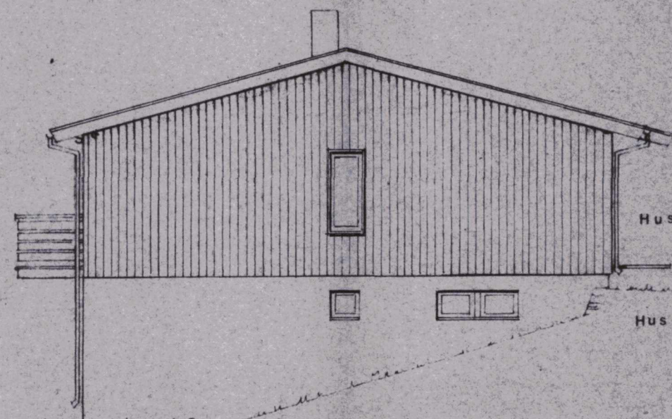
fasade mot sydøst
